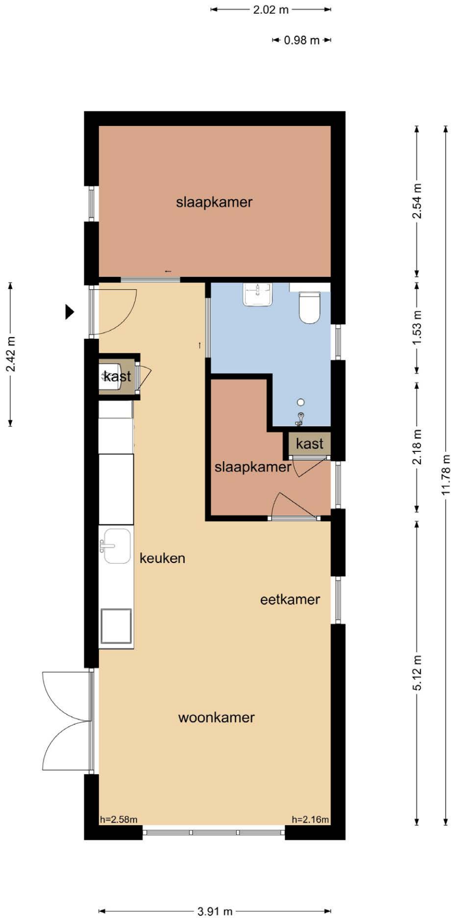
Begane grond
